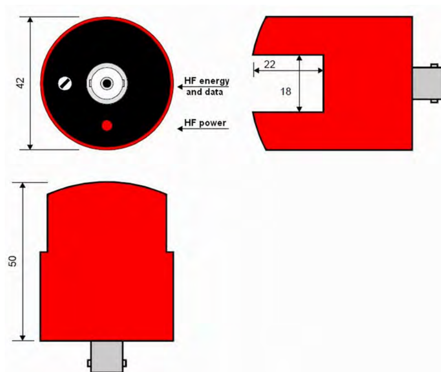
Fig. 4: Stator antenna A8a_PCM
