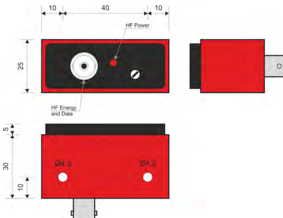
Fig. 4: Stator antenna A8b_PCM
